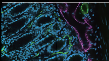
Denoise.ai
