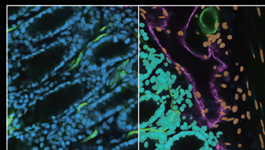
Segment.ai
